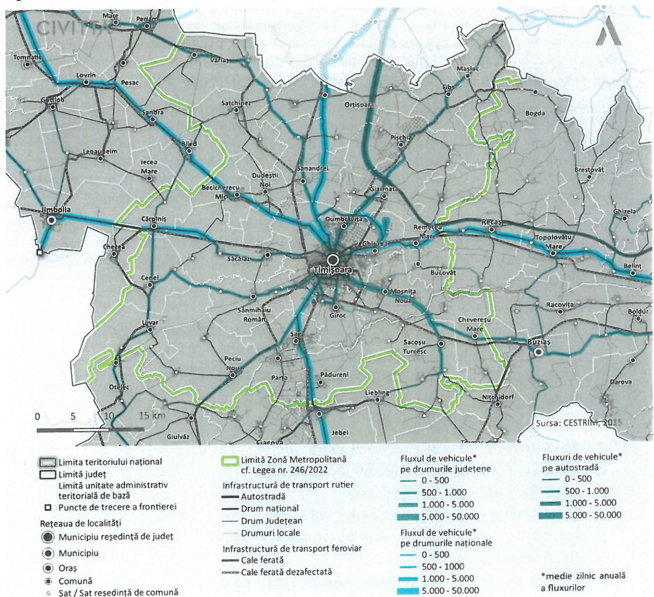
Figura 19 – Volumul de trafic înregistrat pe principalele artere penetrante
