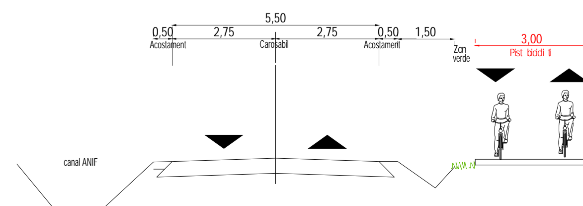
Profil transversal tip 1
