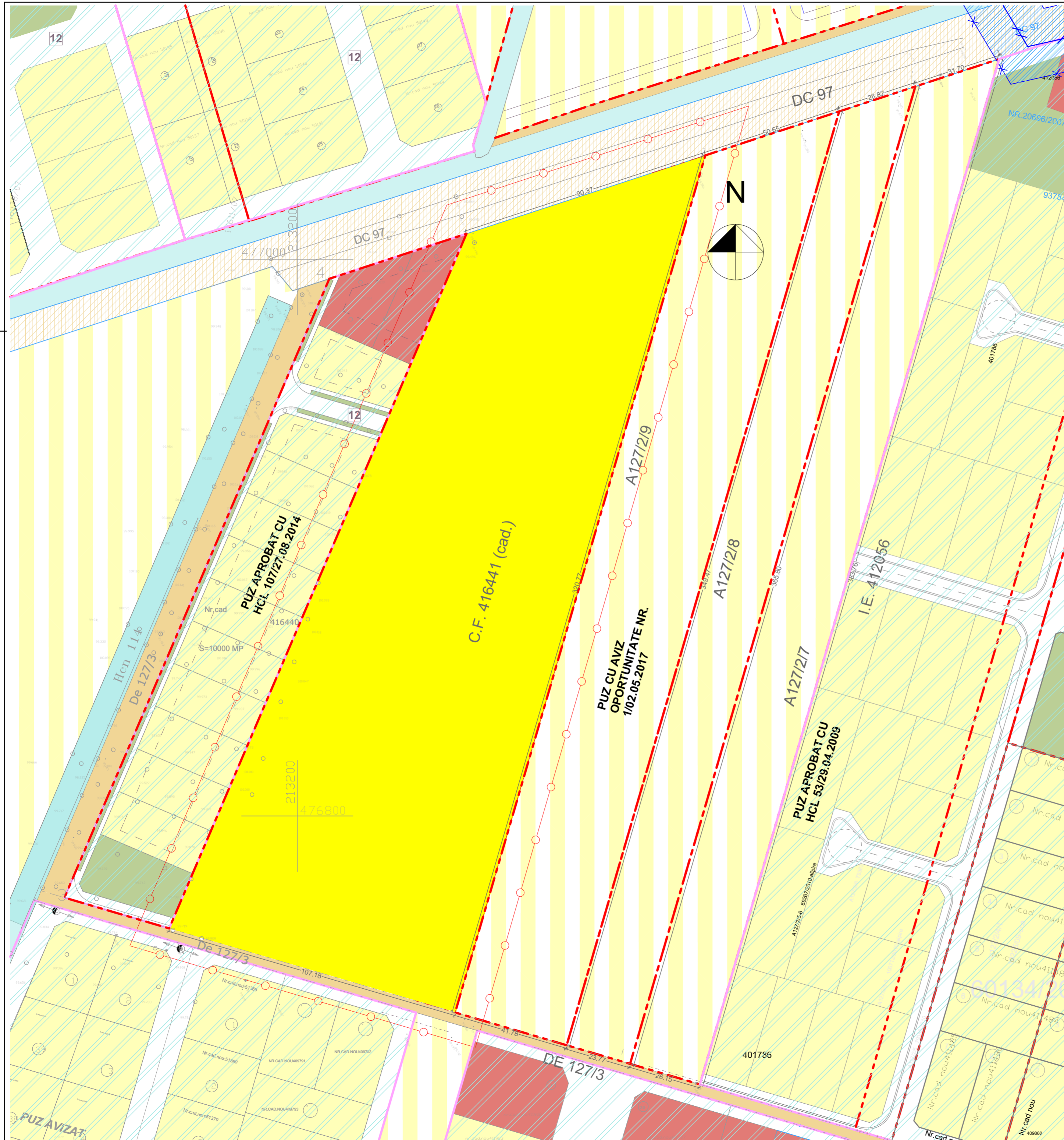
PARCELA AFERENTA PUZ A127/2/10 (cad. 416441) S=26400 m 2
